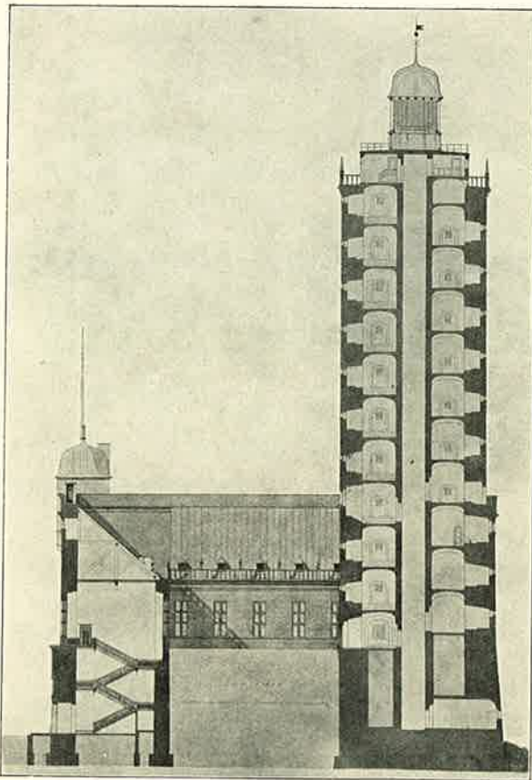
TVÆRSNIT AF TAARN OG TREDJE GAARD.
